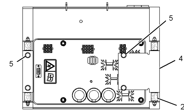
VIEW A-A
